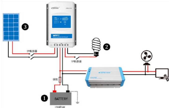
Abb. 2-2 Schaltplan
